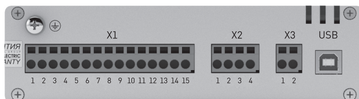
Клеммы CM_16_2
