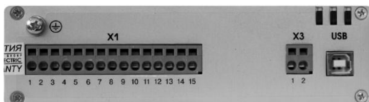
Клеммы CM_16_1
